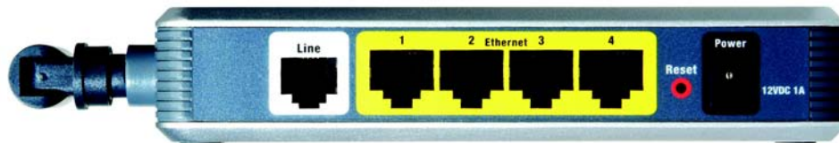
Figure 3-1 : Ports et bouton Reset (Réinitialisation) du panneau latéral
